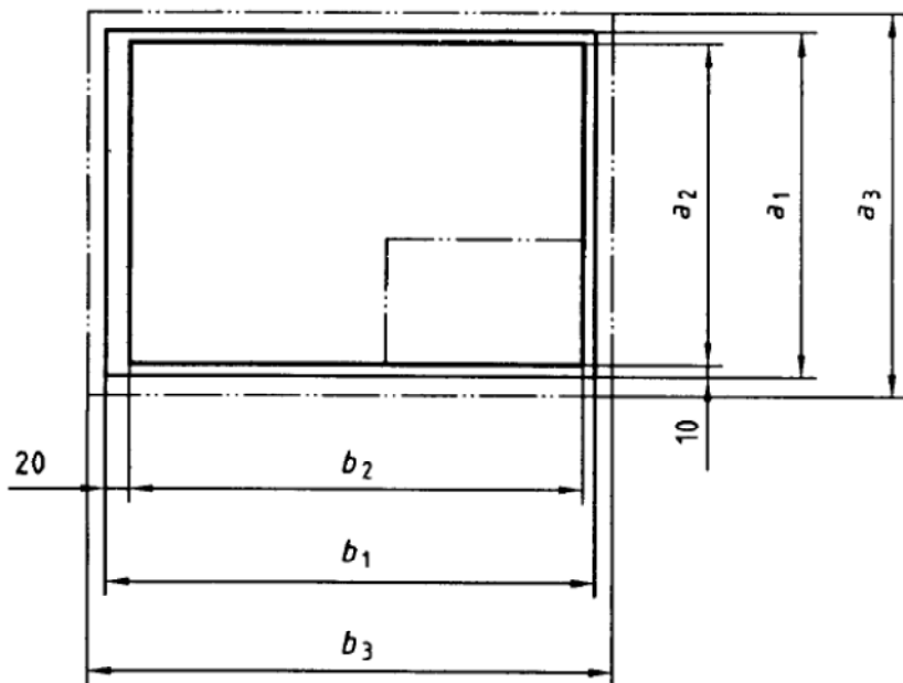
Fig. 1 - Formatos de A3 a A0
